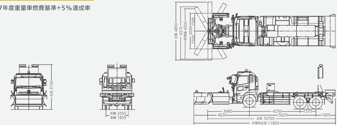
CW 6×4 22t
